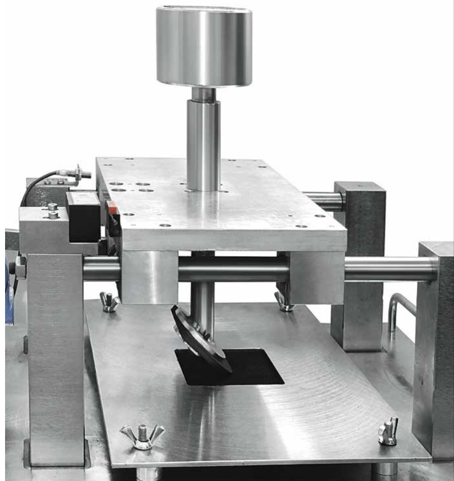
Роботизированное устройство для проведения «испытания каблучком»
